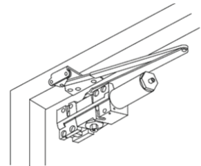
Parallel Arm ชนิดติดแบบขนาน
