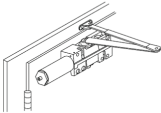
Regular Arm แวนฉากธรรมดา
