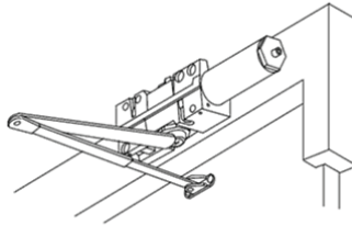
Top Jamb ชนิดติดที่วงกบ
